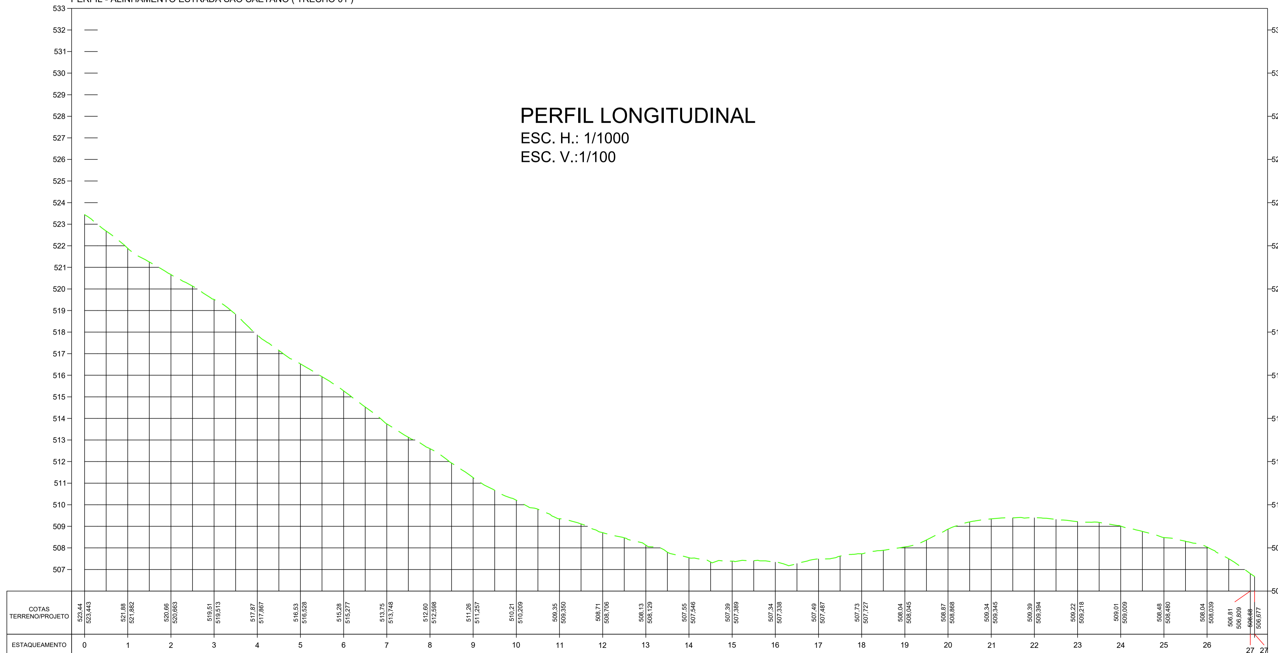
PERFIL - ALINHAMENTO ESTRADA SÃO CAETANO ( TRECHO 01 )
