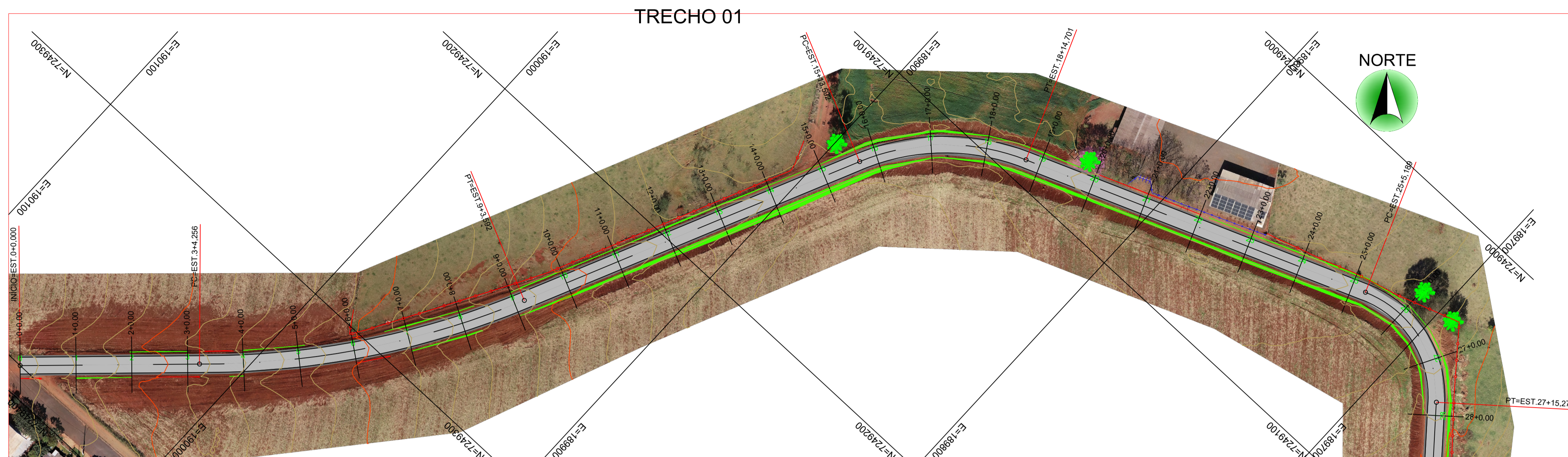
PLANTA BAIXA - GEOMÉTRICO ESC. 1/1000
