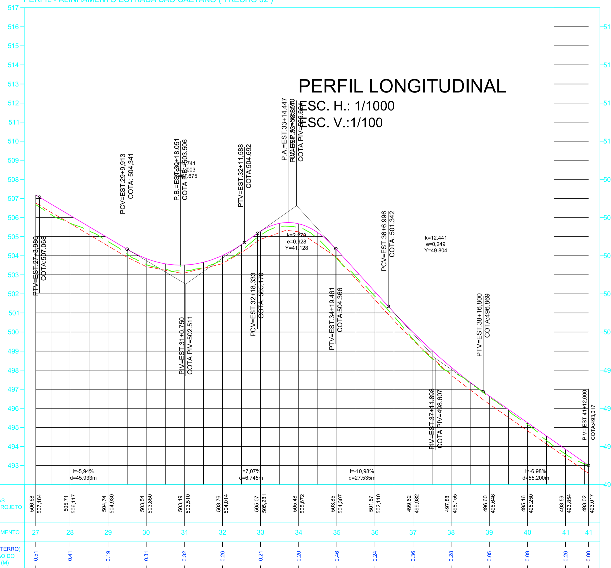
PERFIL - ALINHAMENTO ESTRADA SÃO CAETANO ( TRECHO 02 )
