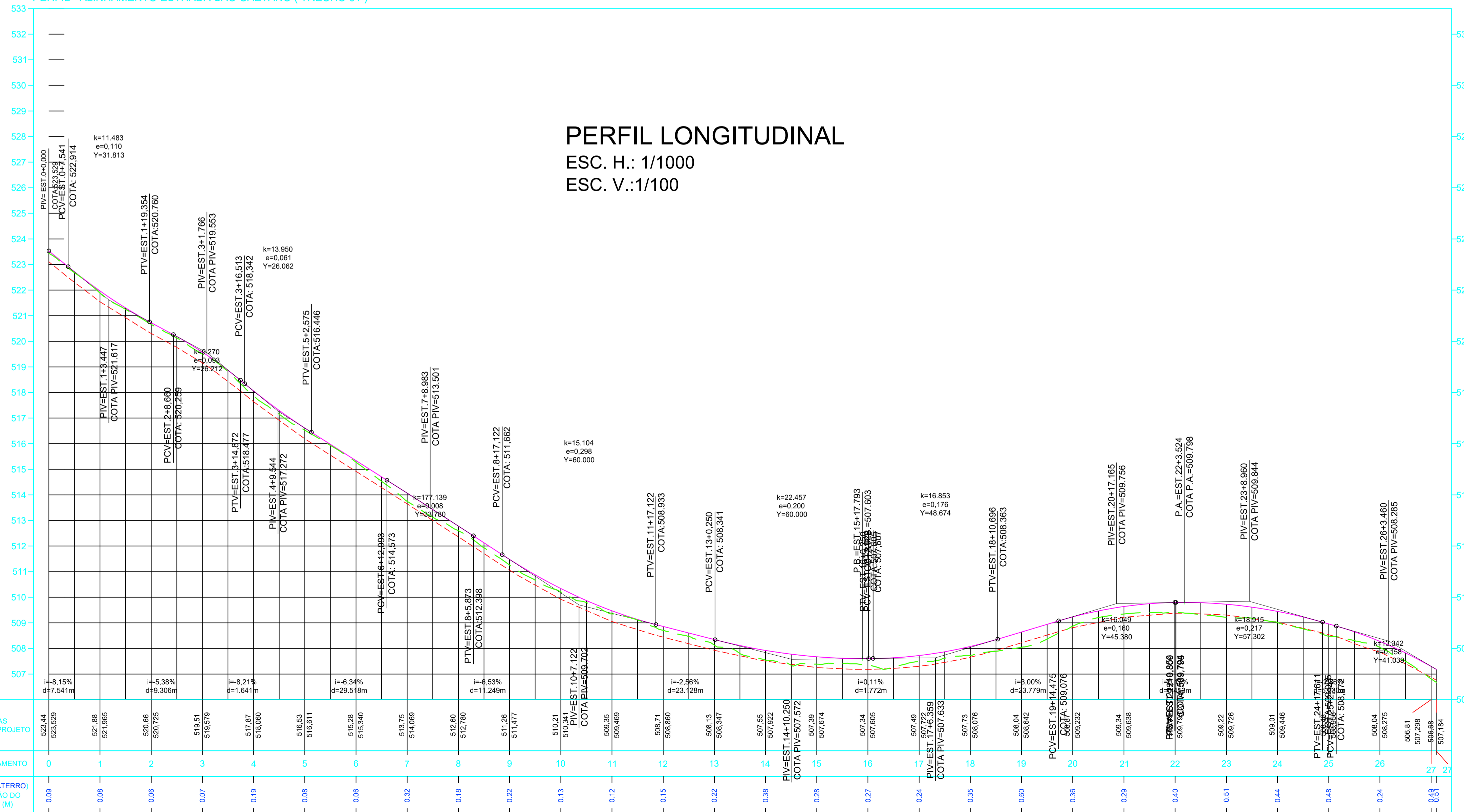
PERFIL - ALINHAMENTO ESTRADA SÃO CAETANO ( TRECHO 01 )
