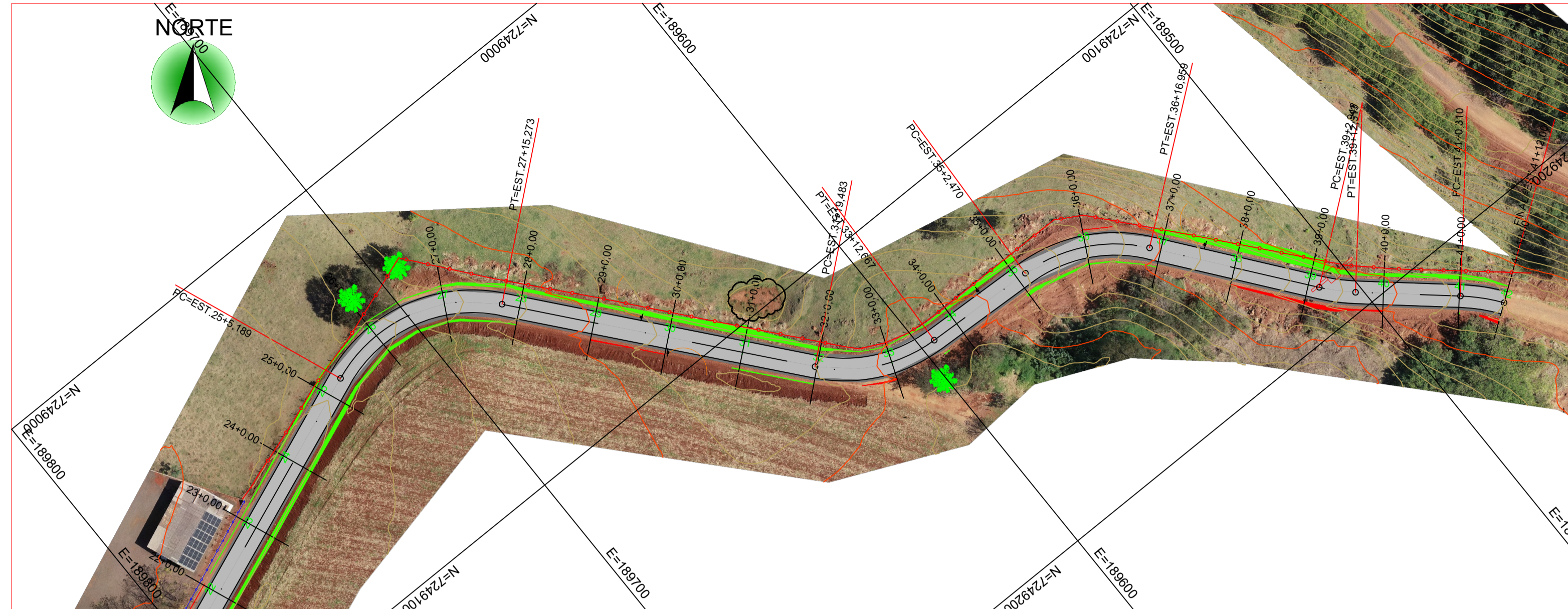
PLANTA BAIXA - GEOMÉTRICO ESC. 1/1000
