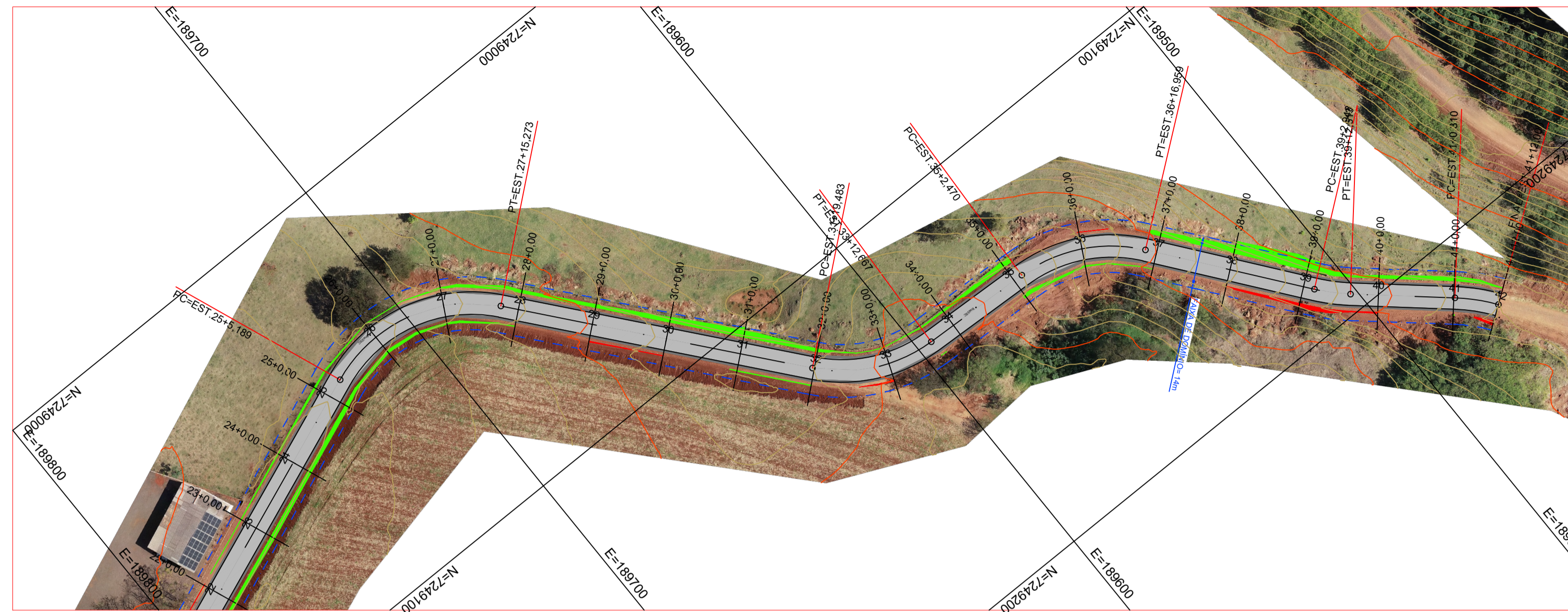
PLANTA BAIXA - TERRAPLENAGEM ESC. 1/1000
